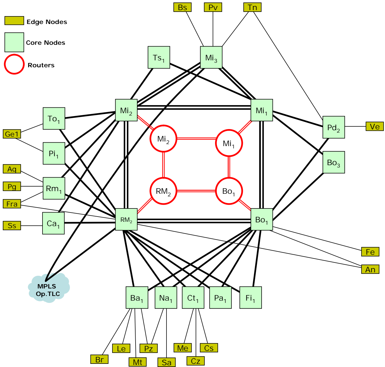
Figura 7: L'infrastruttura di Switching GARR-X
