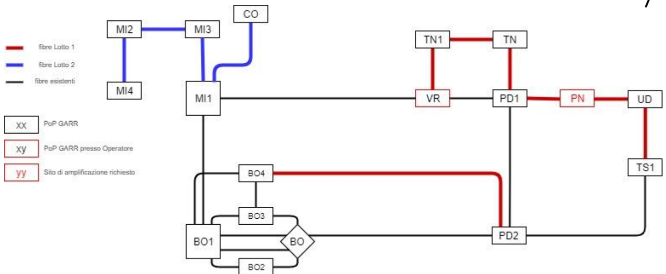
Figura 1: Topologia della rete di dorsale in fibra ottica nell'area interessata all'acquisizione. In nero le tratte già operative, in rosso e blu le tratte di nuova realizzazione oggetto della Fornitura
